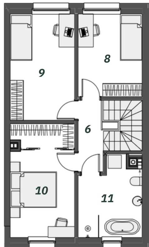
RZUT PIĘTRA
