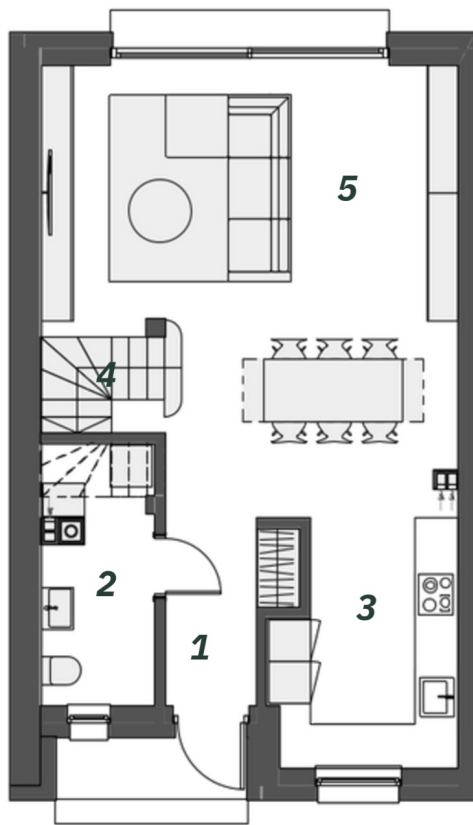
RZUT PARTERU
